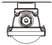
FIG. 5 Fijación a techo o colgada.
